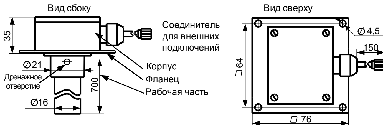
Габаритные и крепежные размеры датчика ДУ-04А
