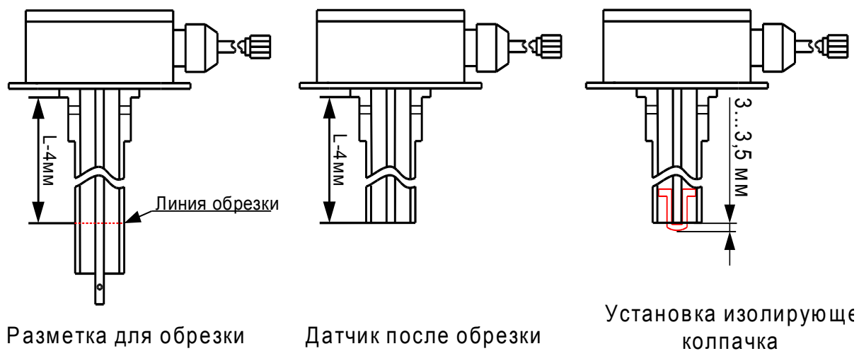
Рис.4 Разметка для обрезки, обрезка датчика до требуемой длины и установка изолирующего колпачка.
